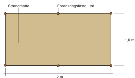
figur 3: I partier utsatta för vågor eller strömmande vatten förankras strandmattan med träspik. Är vågpåverkan kraftig kan förankringen förstärkas ytterligare med hjälp av kokosrep som korsläggs mellan de nedslagna träspikarna.
